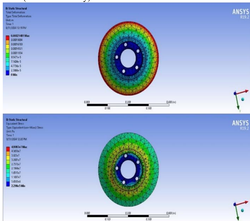
Hình 4: Biến dạng và ứng suất của đĩa phanh hợp kim nhôm
