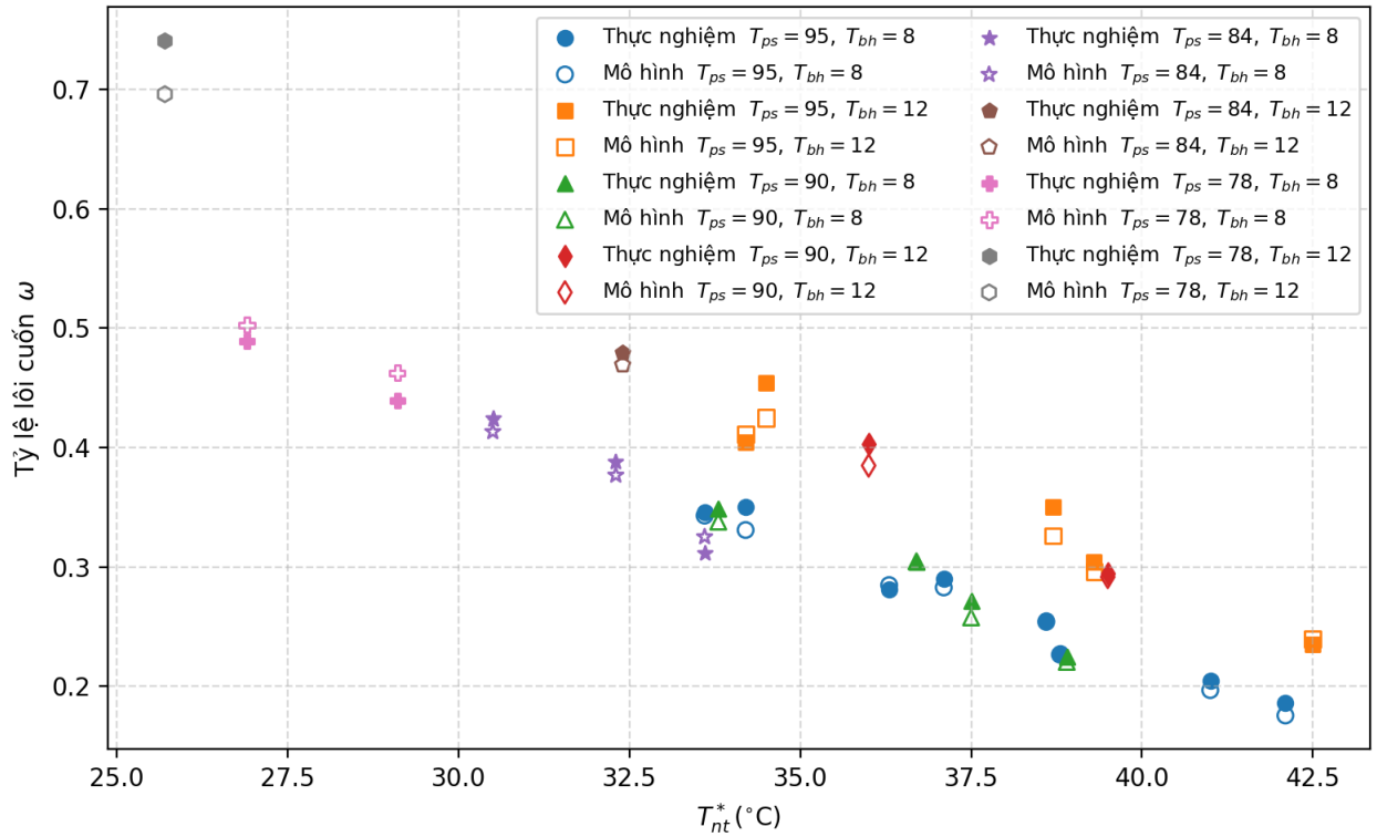
Hình 5a: So sánh tỷ lệ lỗi cuộn của mô hình với thực nghiệm Huang và các cộng sự [5]
