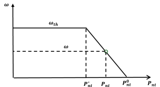
Hình 3: Chế độ dưới tới hạn
