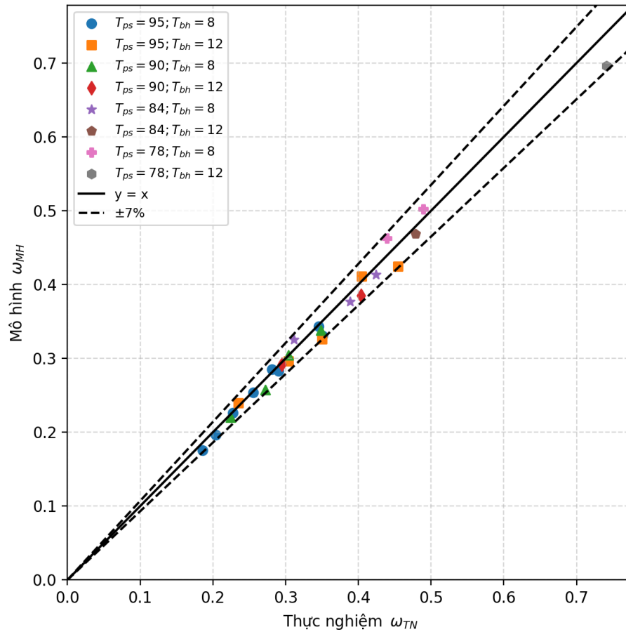
Hình 5b: Sai số giữa mô hình và thực nghiệm của Huang và các cộng sự [5]
