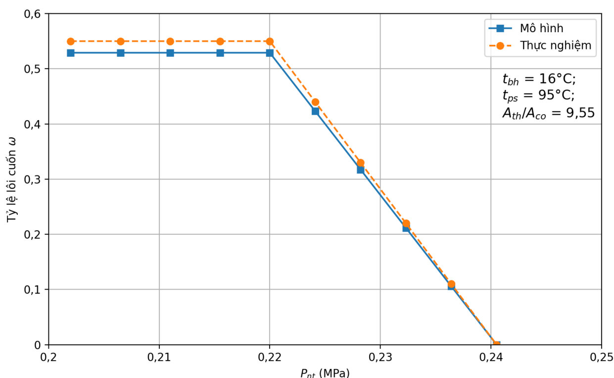
Hình 6: So sánh tỷ lệ lõi cuốn với mô hình của Shestopalov và các cộng sự [12]
