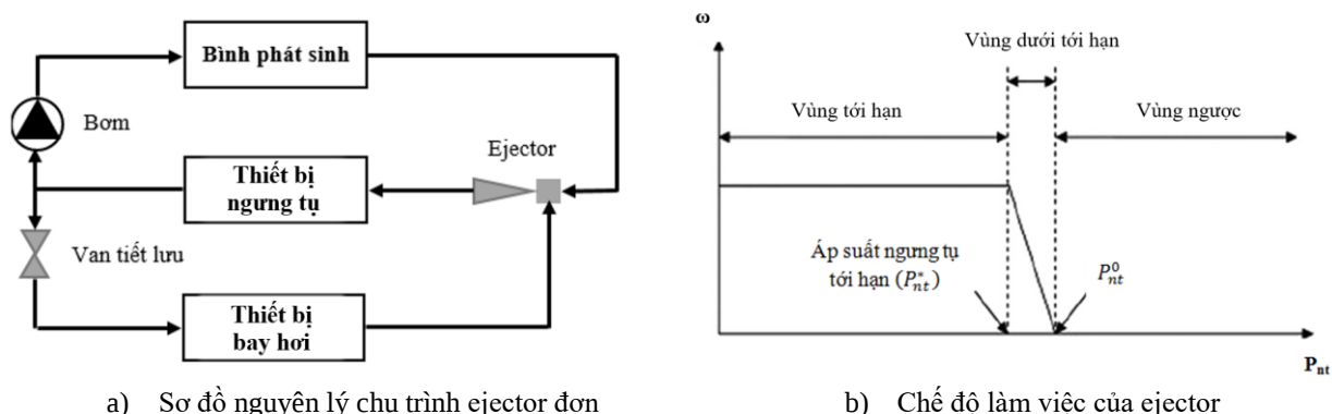
Hình 1: Chu trình ejector đơn và chế độ hoạt động trong ejector
