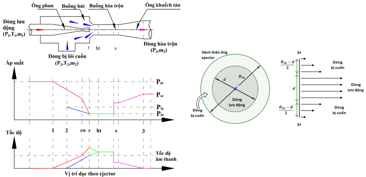
Hình 2: a) Các quá trình trong ejector b) Mặt cắt ht - ht
