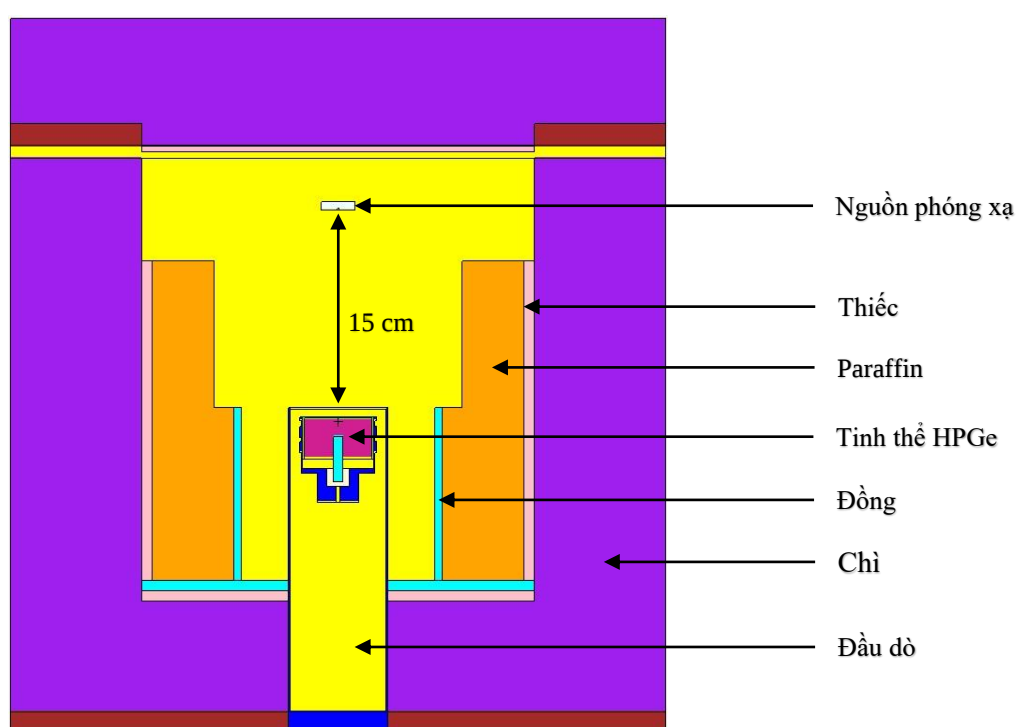
Hình 1. Mặt cắt đứng của buồng chì che chắn phóng bức xạ vẽ bằng chương trình MCNP4C2, được bố trí các lớp vật liệu gồm đồng, paraffin, thiếc, chì tính từ trong ra ngoài và nguồn phóng xạ với thân giữ nguồn làm bằng nhựa epoxy. Trường hợp nguồn đặt cách đầu dò 15 cm.
