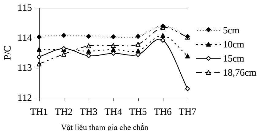
Hình 5. Sự phụ thuộc của tỉ số P/C theo vật liệu tham gia che chắn và theo khoảng cách nguồn - đầu dò.
