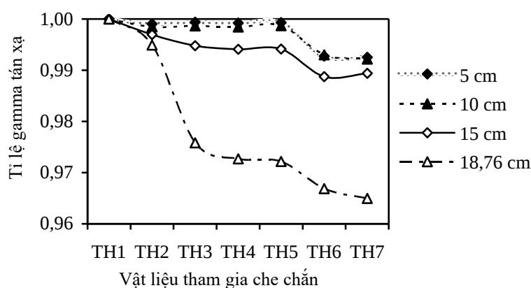
Hình 4. Tỉ lệ gamma tán xạ ở miền tán xạ Compton theo vật liệu tham gia che chắn và theo khoảng cách nguồn - đầu dò.
