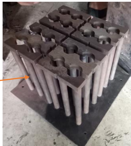
Hình 30: Khuôn đực
