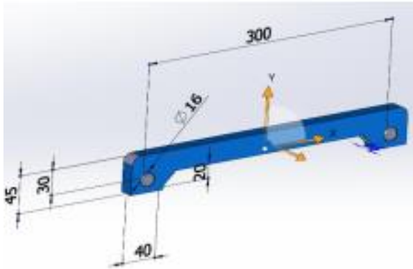
Hình 20: Thiết kế thanh đỡ
